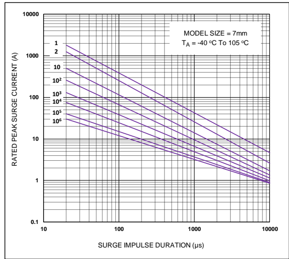
CNR-07V201K to CNR-07V821K
