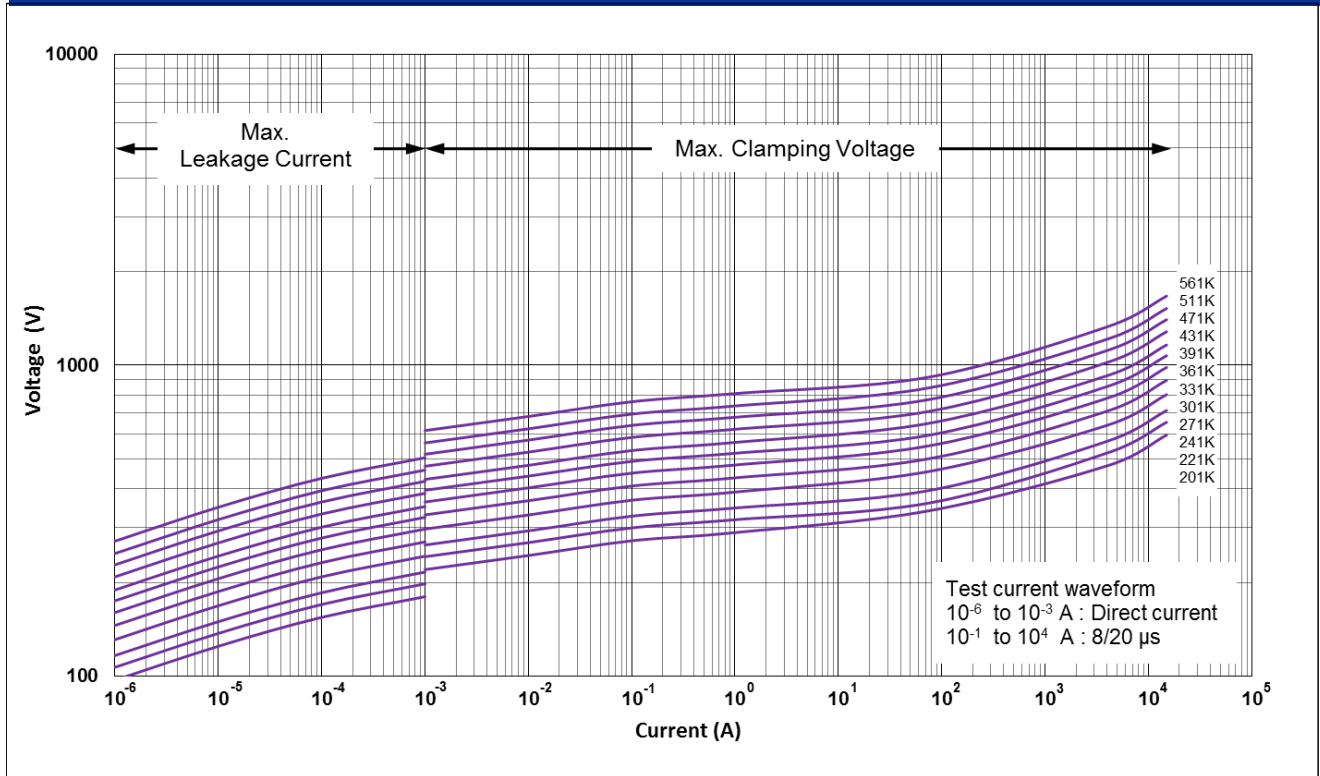
CNR-18N201K to CNR-18N561K V-I Curves
