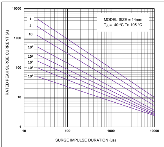
CNR-14D781K to CNR-14D182K
